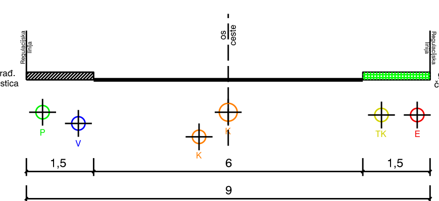
PRESJEK 2-2
