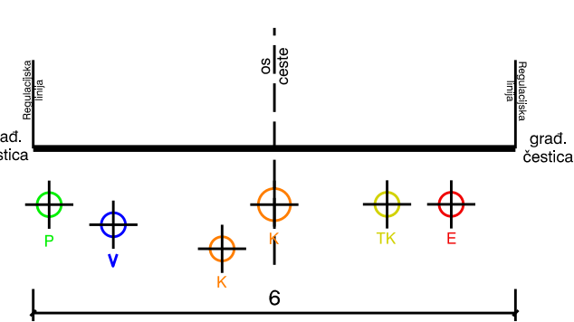
PRESJEK 1-1
