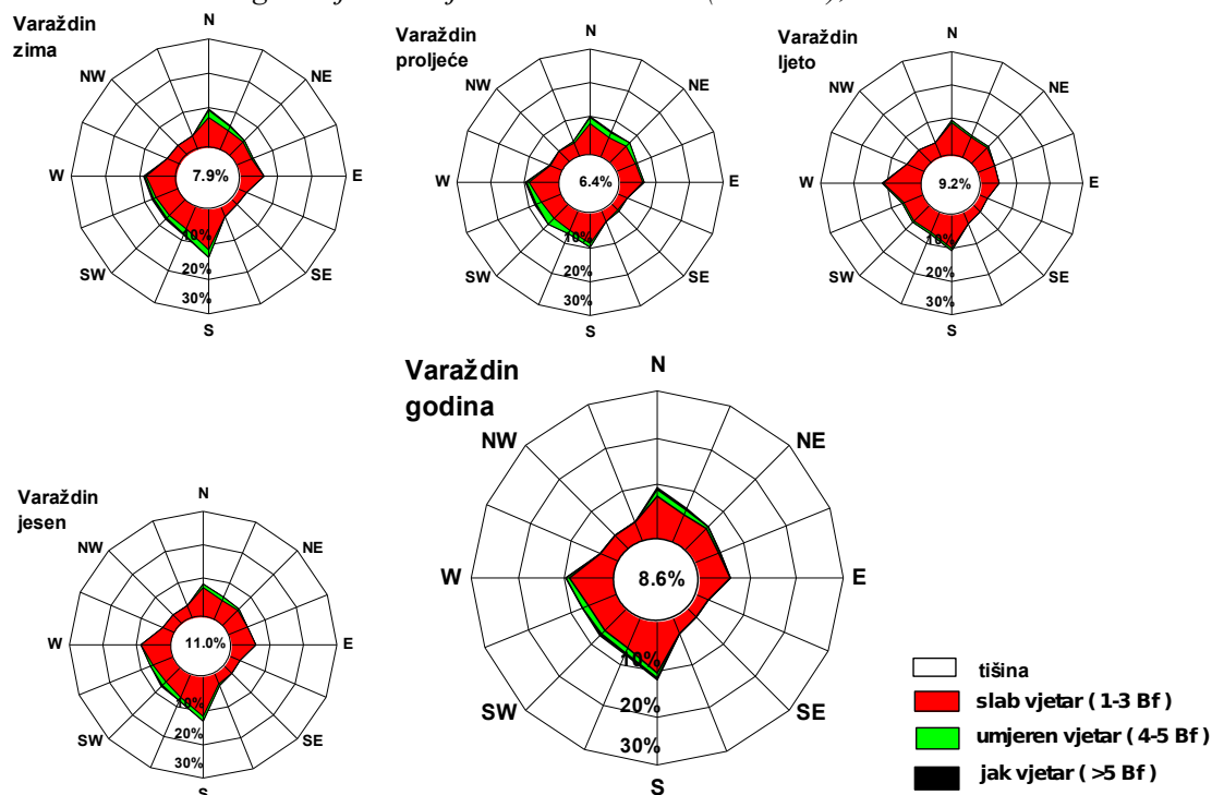
Slika 2: Sezonske i godišnja ruža vjetrova za Varaždin (Breznicu), 1981.-2000.
